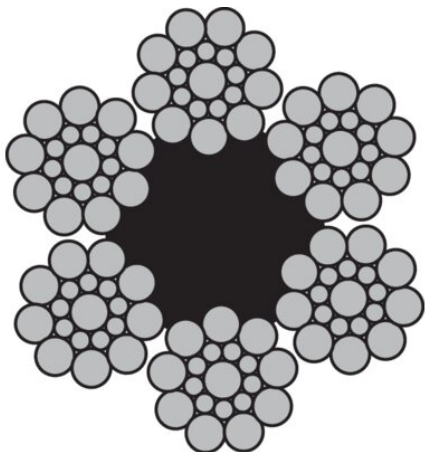
Teräsköysiraksi
